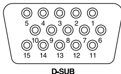
D-SUBミニ15ピンコネクタ
