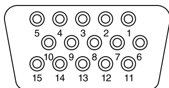
D-SUB
