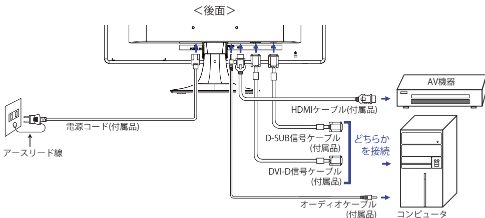
[ 接続例 ]
