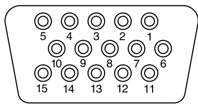
D-SUB
