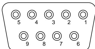
D-SUB
